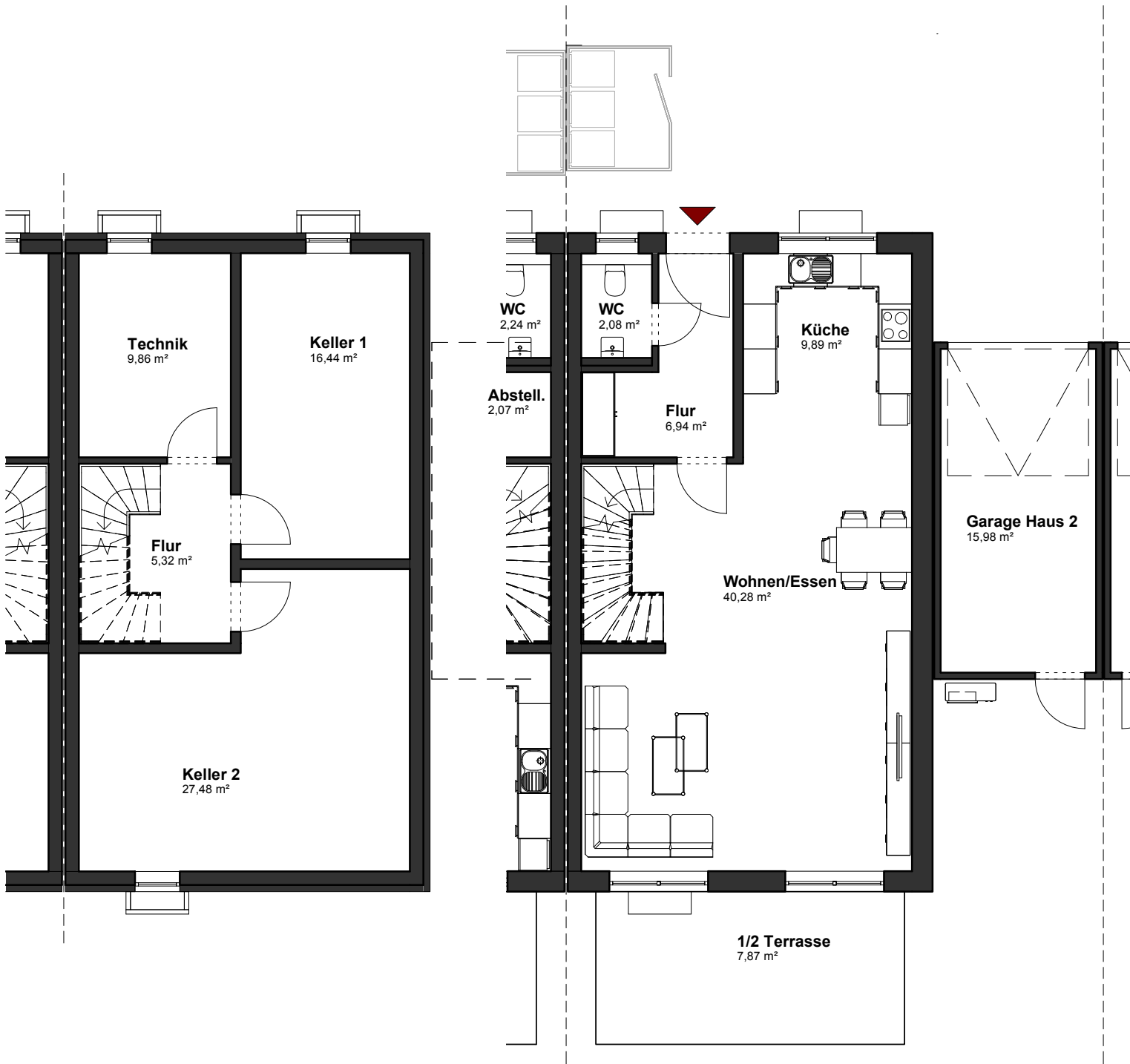
Haus 2 Kellergeschoss
