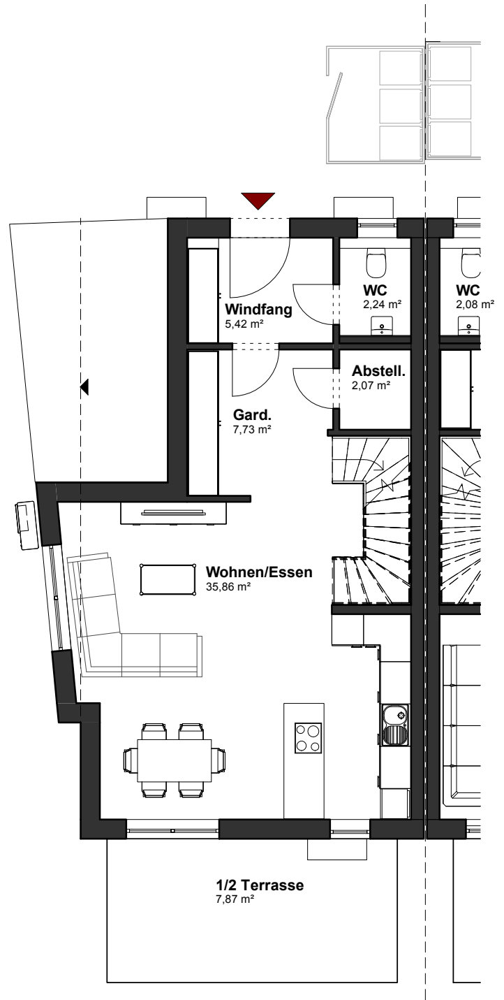
Haus 1 Erdgeschoss
